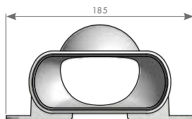
Raccord mixte plat - rond Ø80mm
