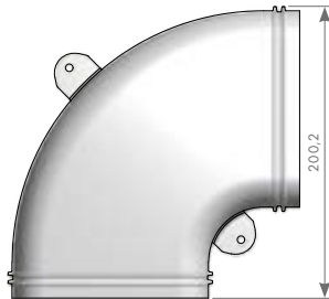
Courbe horizontale 90°
