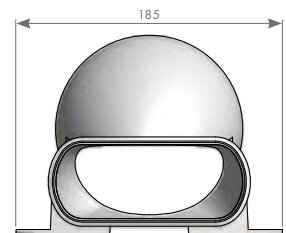
Raccord mixte plat - rond Ø125mm
