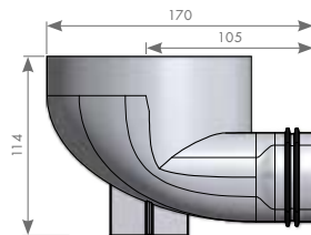
Courbe horizontale 90°
