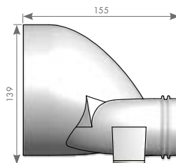
Raccord mixte plat - rond Ø125mm
