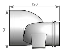
Raccord mixte plat - rond Ø80mm
