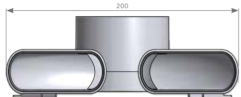
Raccord double pour grille d'extraction Ø125mm
