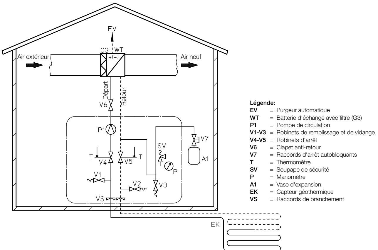
■ Fig. 3 - Raccordement hydraulique
