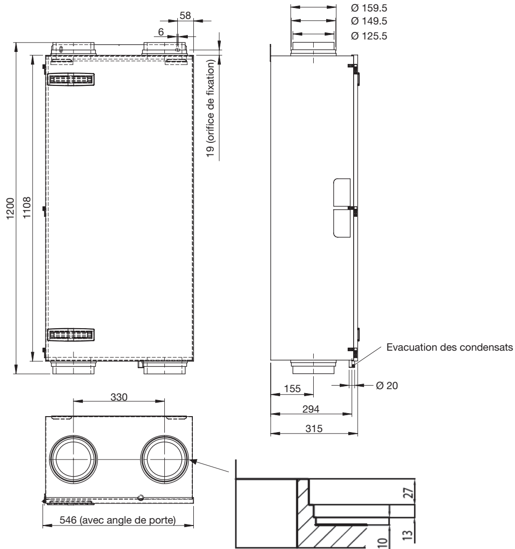
Schémas cotés (variante à droite)
