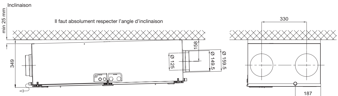
Schémas cotés (montage au plafond)
